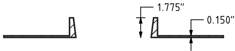
SECTION A-A
