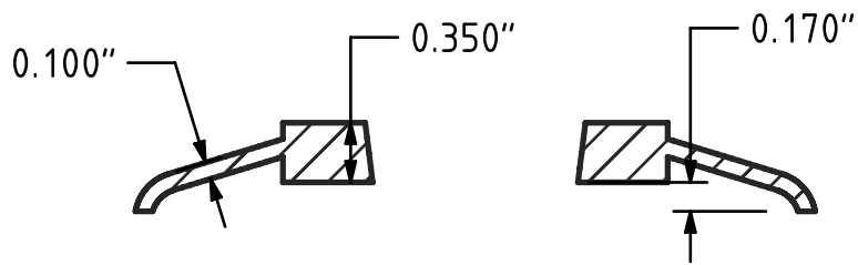
SECTION A-A
